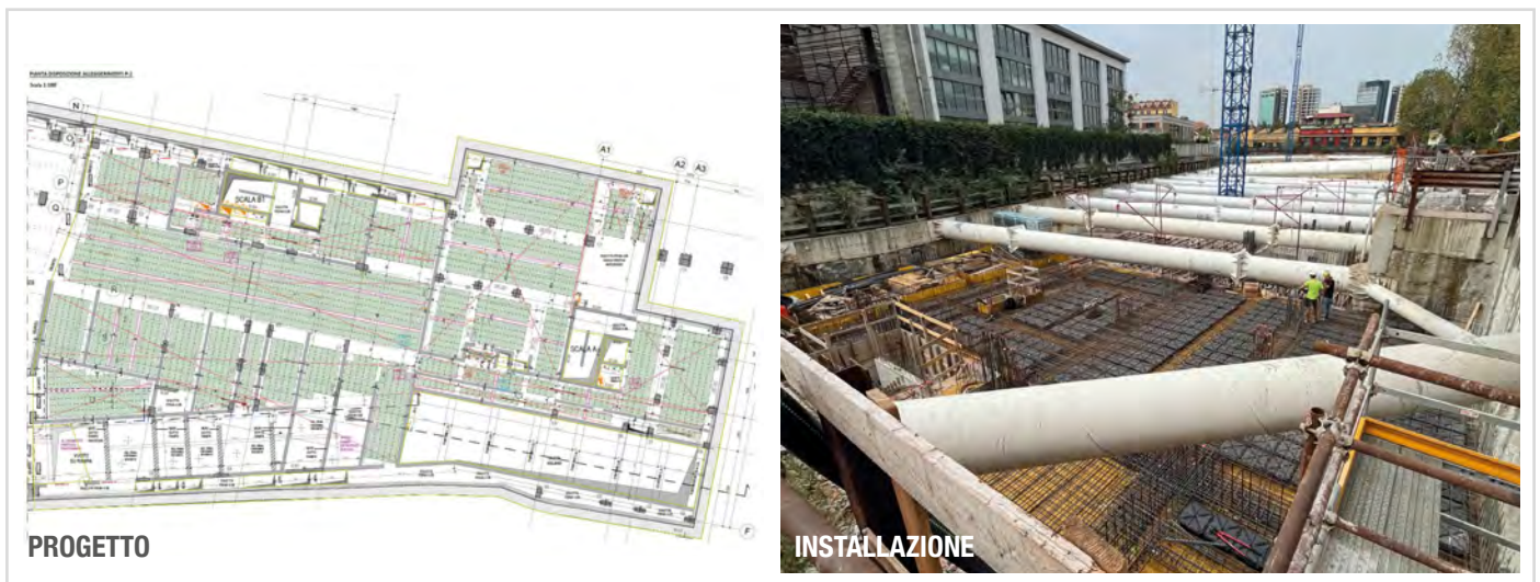
Edificio multipiano a Milano, Italia
