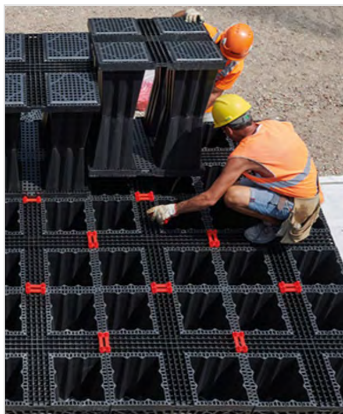
Montaggio Aquabox
