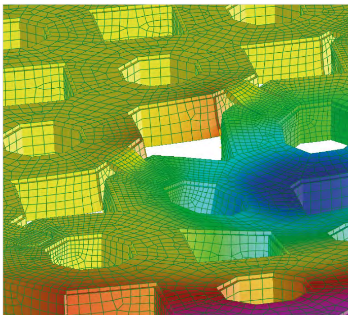
Analisi di deformazione del modello FEM Geocross
