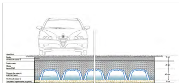
Stratigrafia vasca tipo Aquabox
