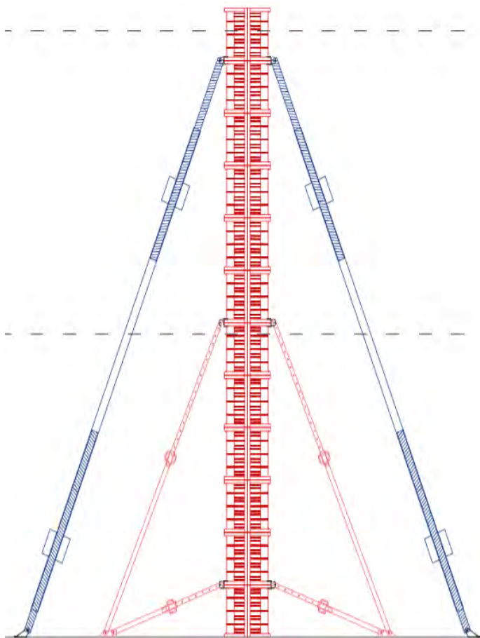
Schema sistema di cassetta
