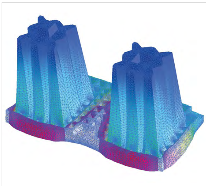
Analisi di deformazione del modello FEM Aquabox
