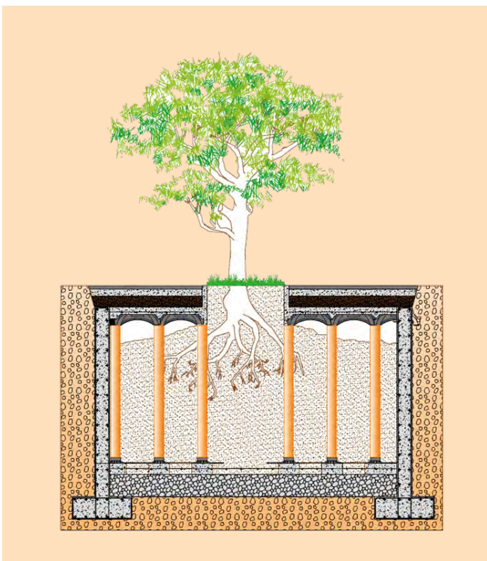
Sezione Elevator Root
