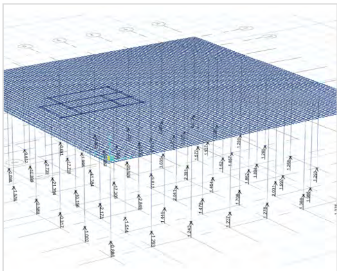
Modello di calcolo, Pacific Center, Panama
