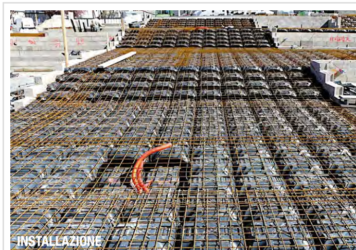
Cantiere Elevator per la Gare de Sarchelle, Francia
