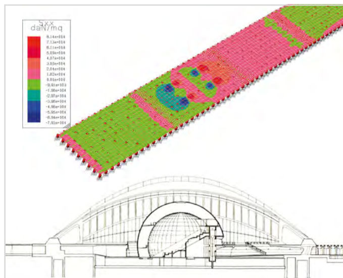
Analisi FEM, Elevator per Expo 2020, Dubai
